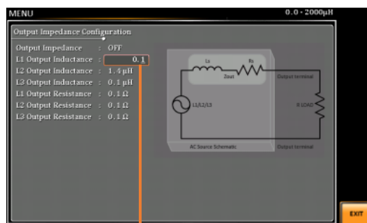
L1 出カインダクタンス設定
