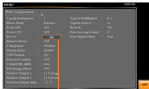
Buzzer 設定
