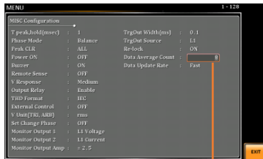
Data Average Count 設定
