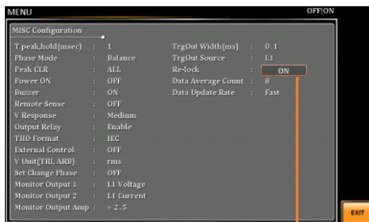
Re-lock 設定
