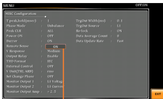
Remote Sense 設定
