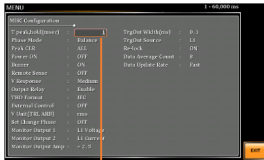
Tpeak,Hold 設定
