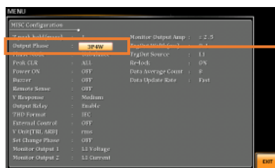
出力相選択
